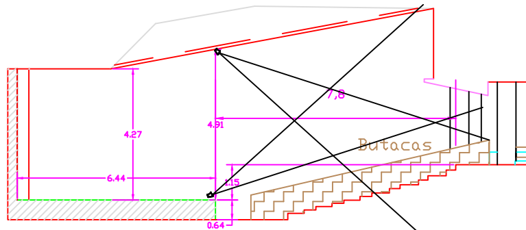
SECCION AB
